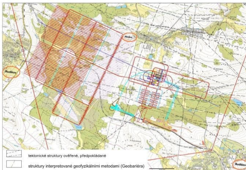
Podzemní stavby hlubinného úložiště
